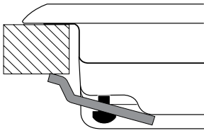
Монтаж крюка для опорных брусков H=20\text{мм}
