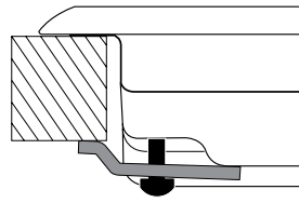
Монтаж крюка для опорных брусков H=30\text{мм}
