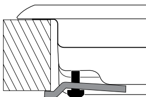
Монтаж крюка для опорных брусков H=40\text{мм}
